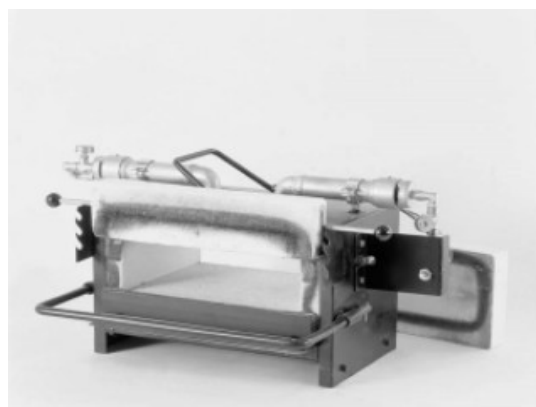
dvojno izgorevanje 1559/2 est. 410x255x255mm int. 300x250x90mm 1150,00 EUR/kos
